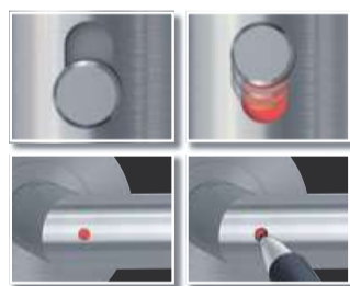
Smart2Lock-Verriegelung ohne Schlüssel- oder WC-Rosetten. Roter Punkt außen zeigt ob Tür verriegelt ist. Not-Entriegelung durch Eindrücken.
