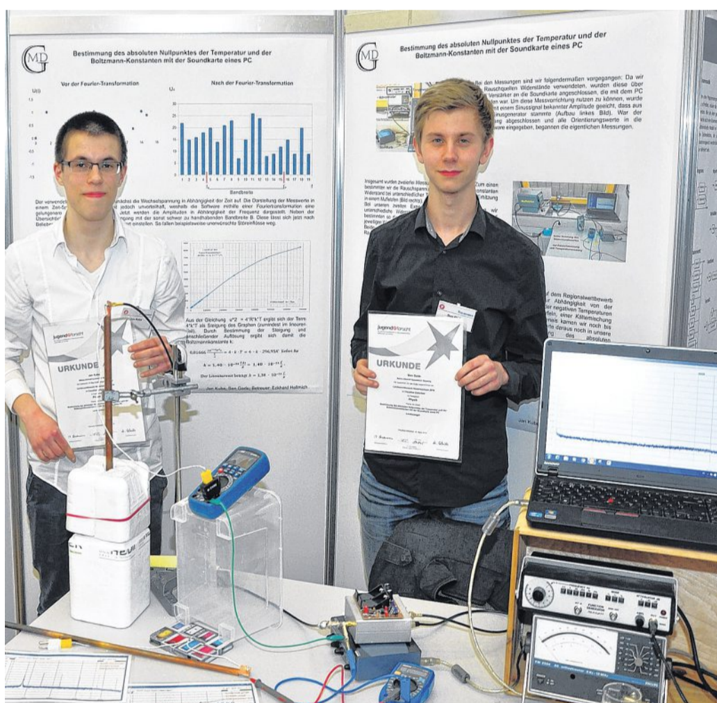
Jan Kube und Ben Gade mit ihren Siegerurkunden in der Aula der Universität Clausthal-Zellerfeld. Im Vordergrund links die Thermobox, in der mit Trockeneis bei -65°C das Rauschen eines Widerstandes gemessen wird. Das Messgerät ist dabei eine hochwertige Soundkarte und ein PC, der das Spektrum der Rauschspannung anzeigt. Marion-Dönhoff-Gymnasium (3)
